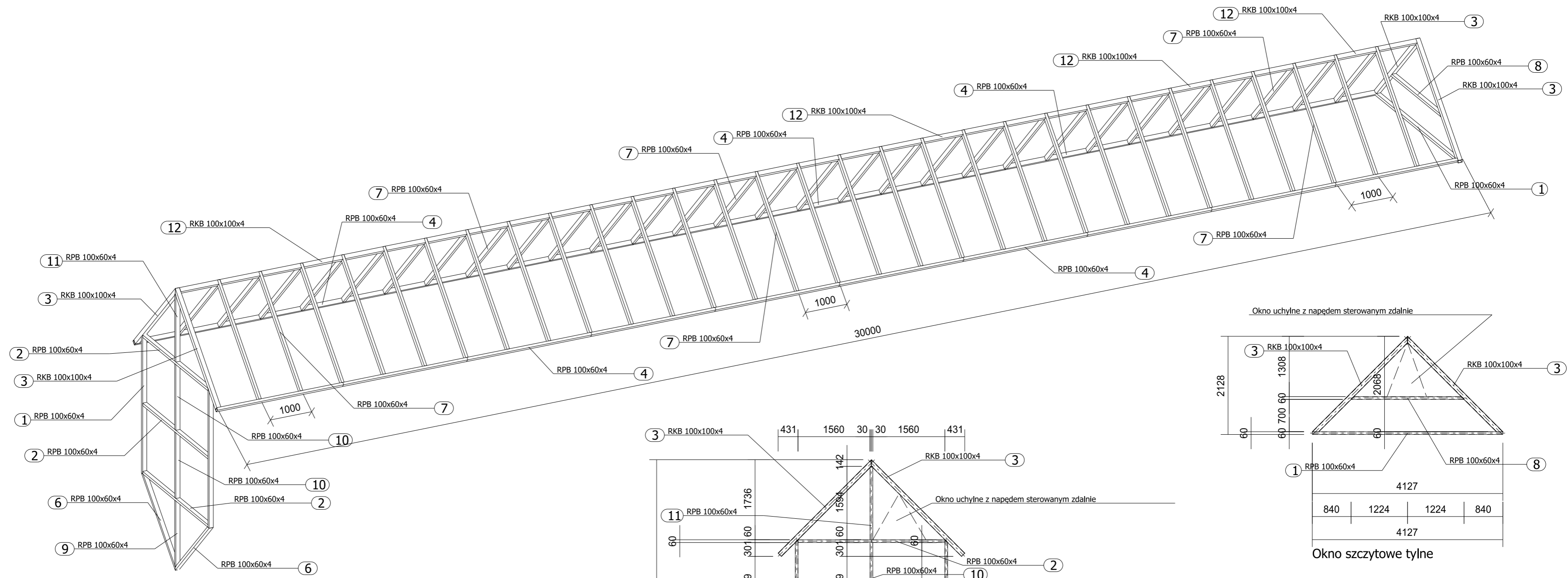
Świetlik Widok
